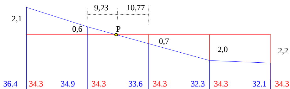
Figura 27 – Perfil seção B.
