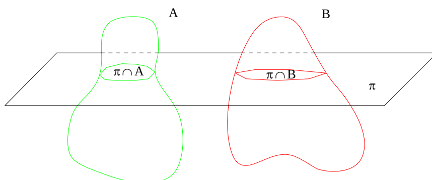
Figura 3 – Princípio de Cavalieri (Adaptada de LIMA, 1975, p.50).
