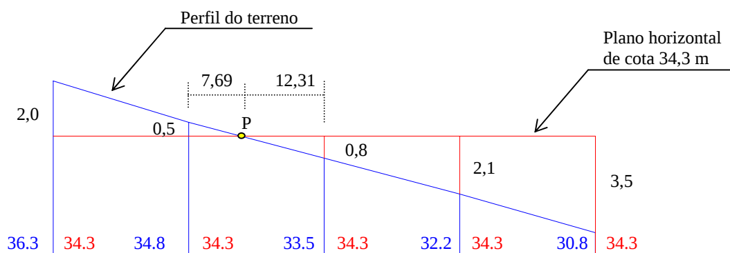
Figura 26 – Perfil seção A.
