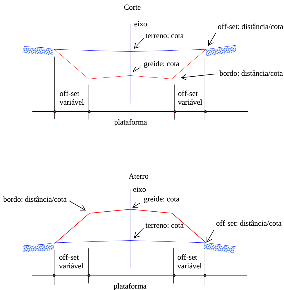
Figura 20 – Nomenclatura das seções transversais.
