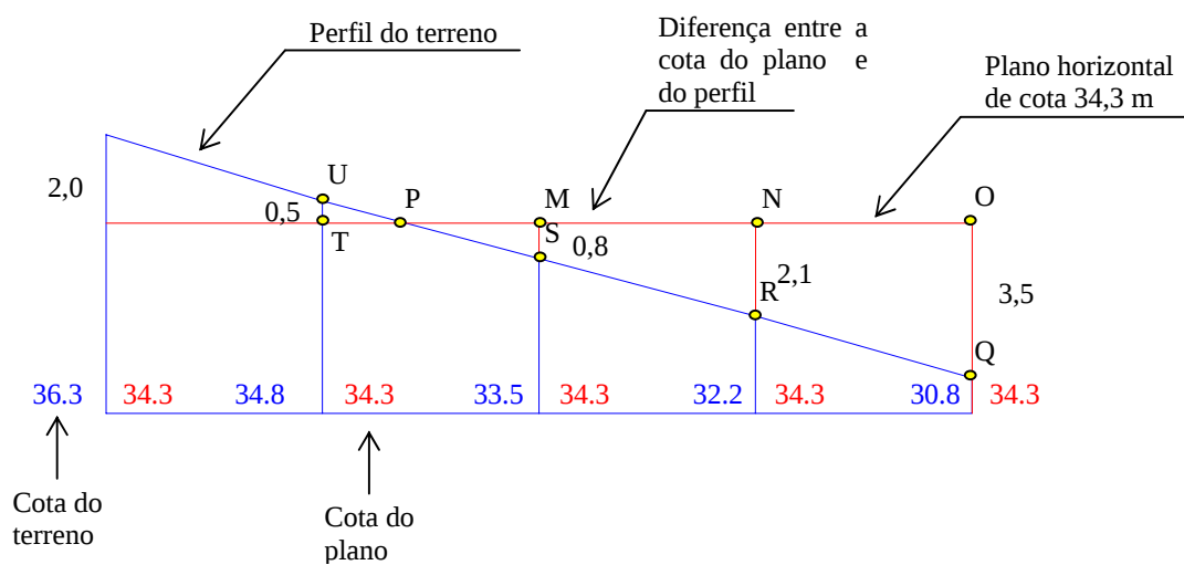
Figura 24 – Perfil “A” do terreno.
