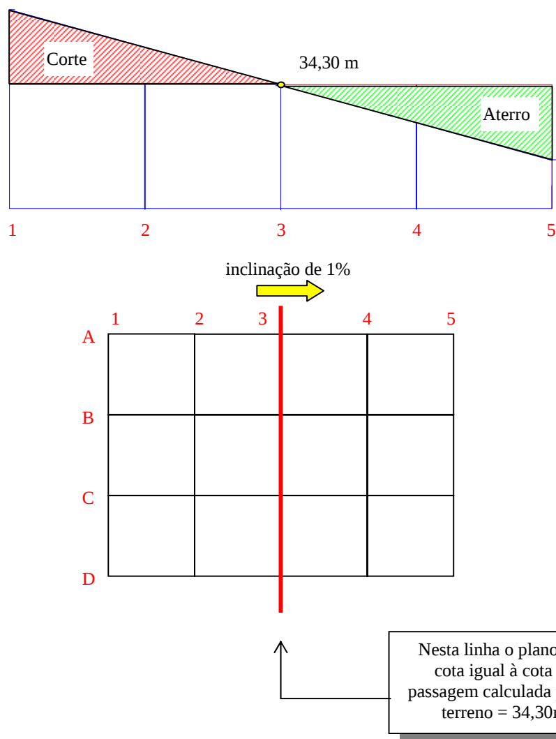
Figura 32 – Posicionamento do plano na hipótese 03.
