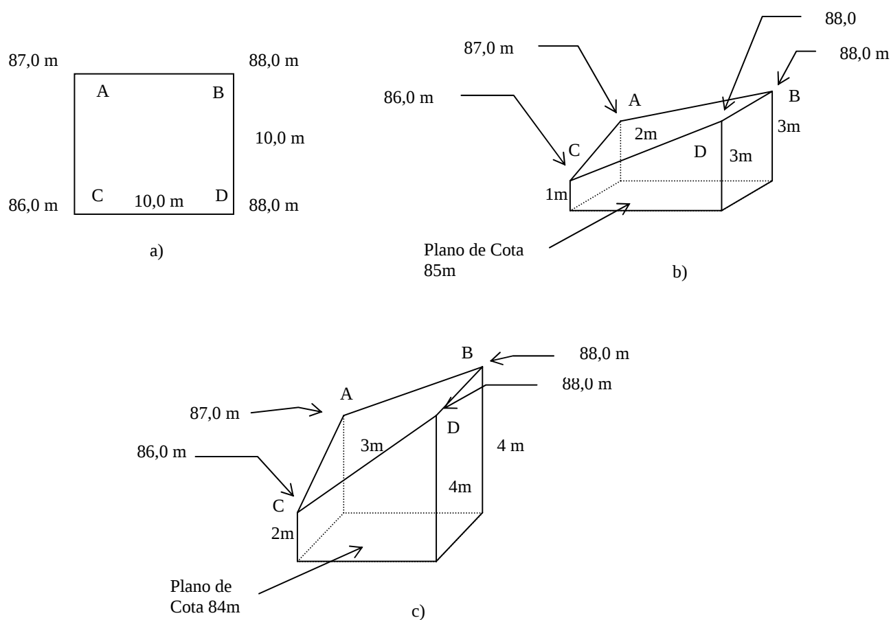
Figura 9 – Volume pelo método das alturas ponderadas.
