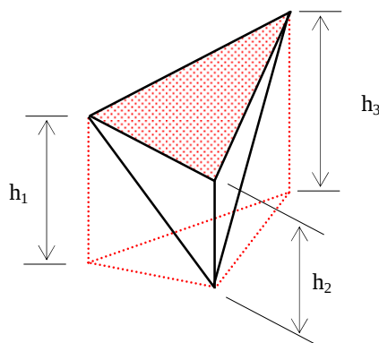
Volume de um tronco de prisma triangular
