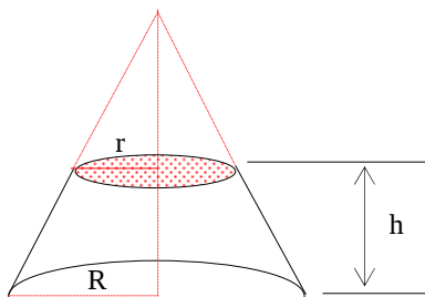
Volume de um tronco de cone
